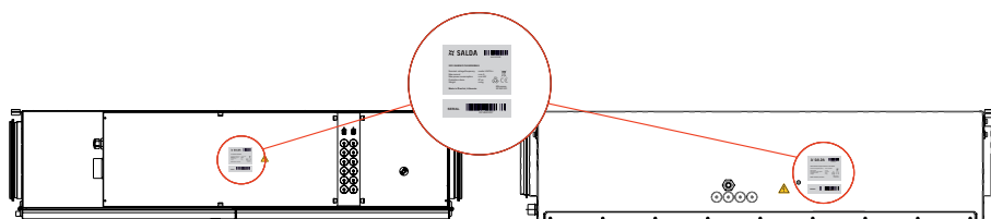
Рис. 2.2. Место технической этикетки на RIS V EKO 3.0
