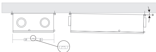
Рис. 13.1. RIS 700 V EKO 3.0 позиция монтажа ( \alpha > 1^\circ )
