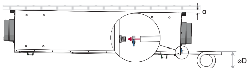
Рис. 13.1.2. установка дренажа ( \varnothing D = 150 \text{ mm} )
